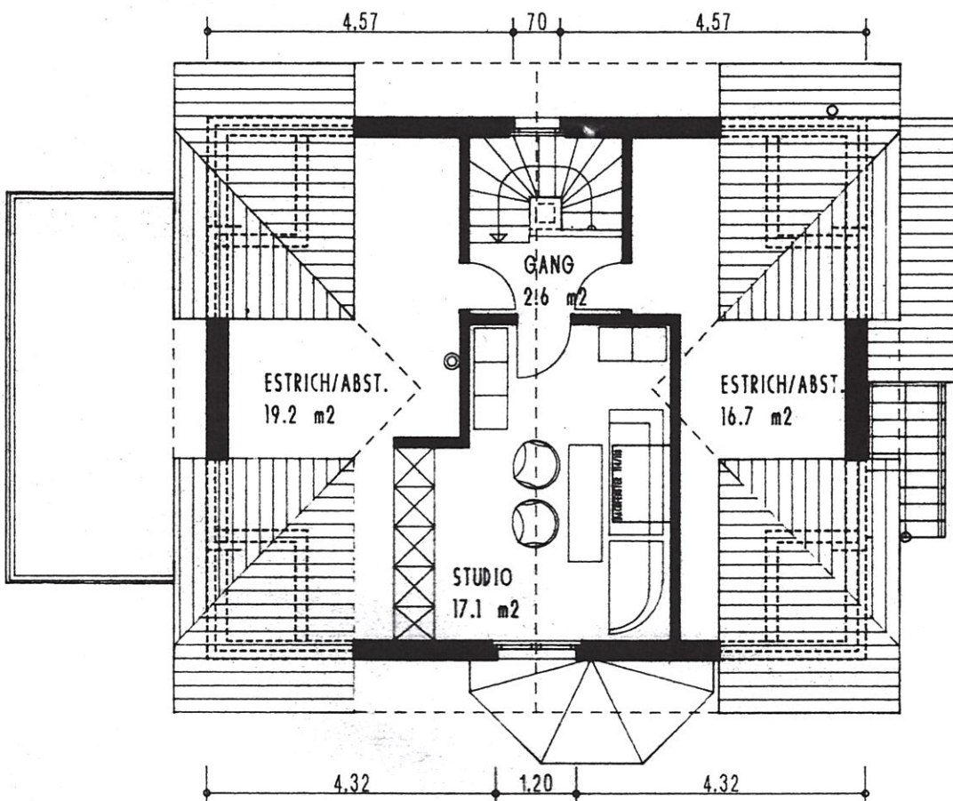
DACHGESCHOSS MST. 1:100
