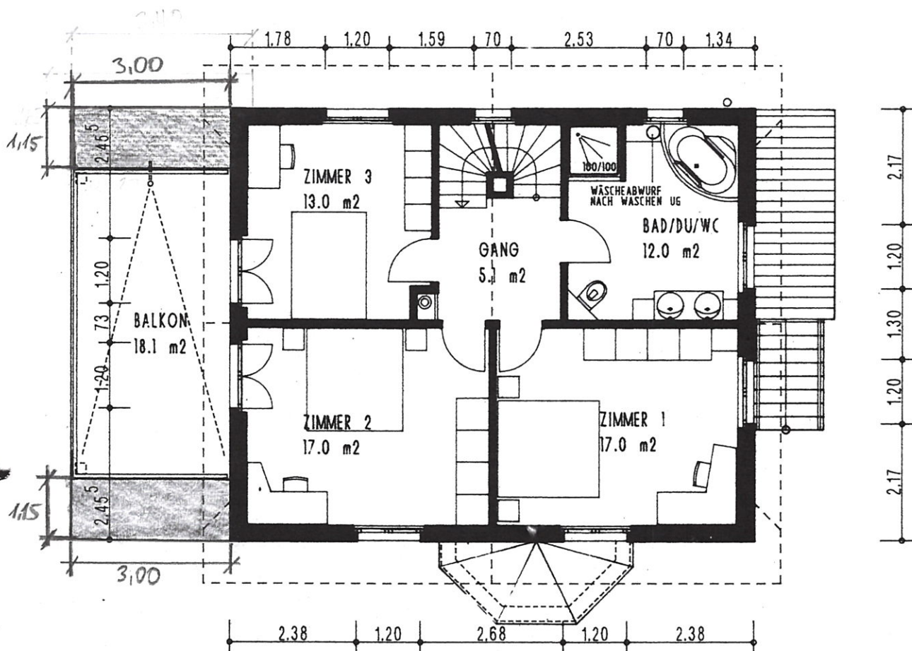
OBERGESCHOSS MST. 1:100
