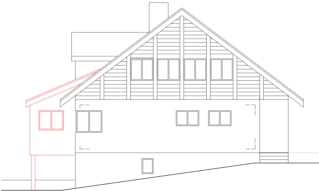
Ost-Fassade
