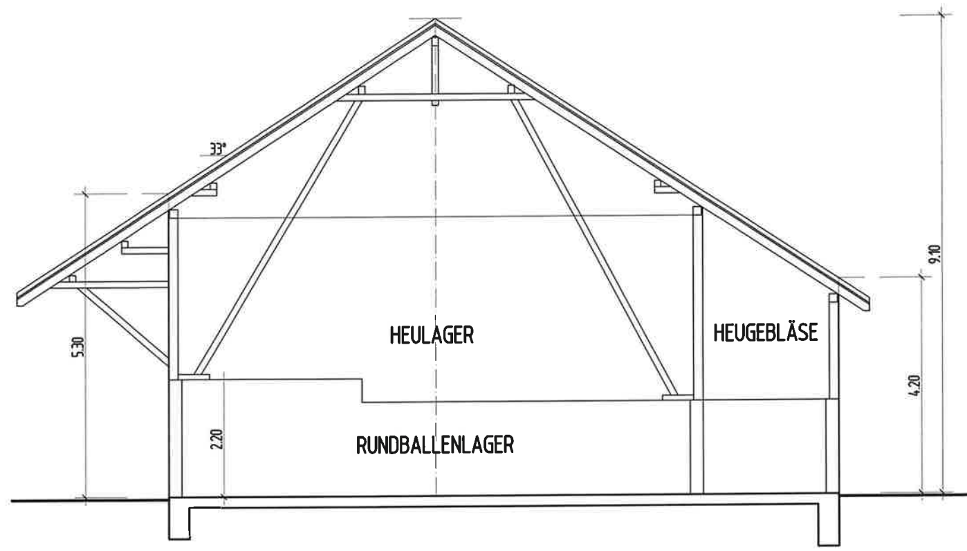
SCHNITT. A-A
